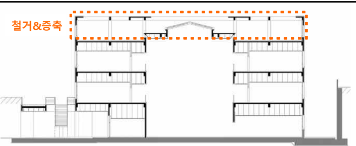
봉안당 증축(안) 단면도
